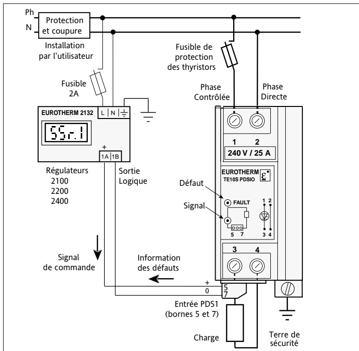
Exemple de branchement du TE10S (entrée PDS1) et du régulateur Eurotherm 2132 (configuration SSr.1)
